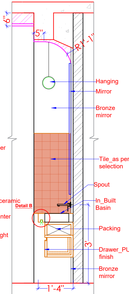
ELEVATION - b
