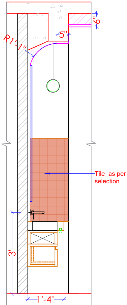
ELEVATION - c
