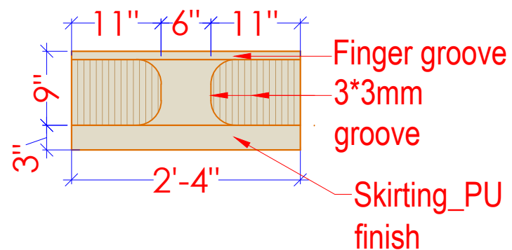
SIDE TABLE ELEVATION
