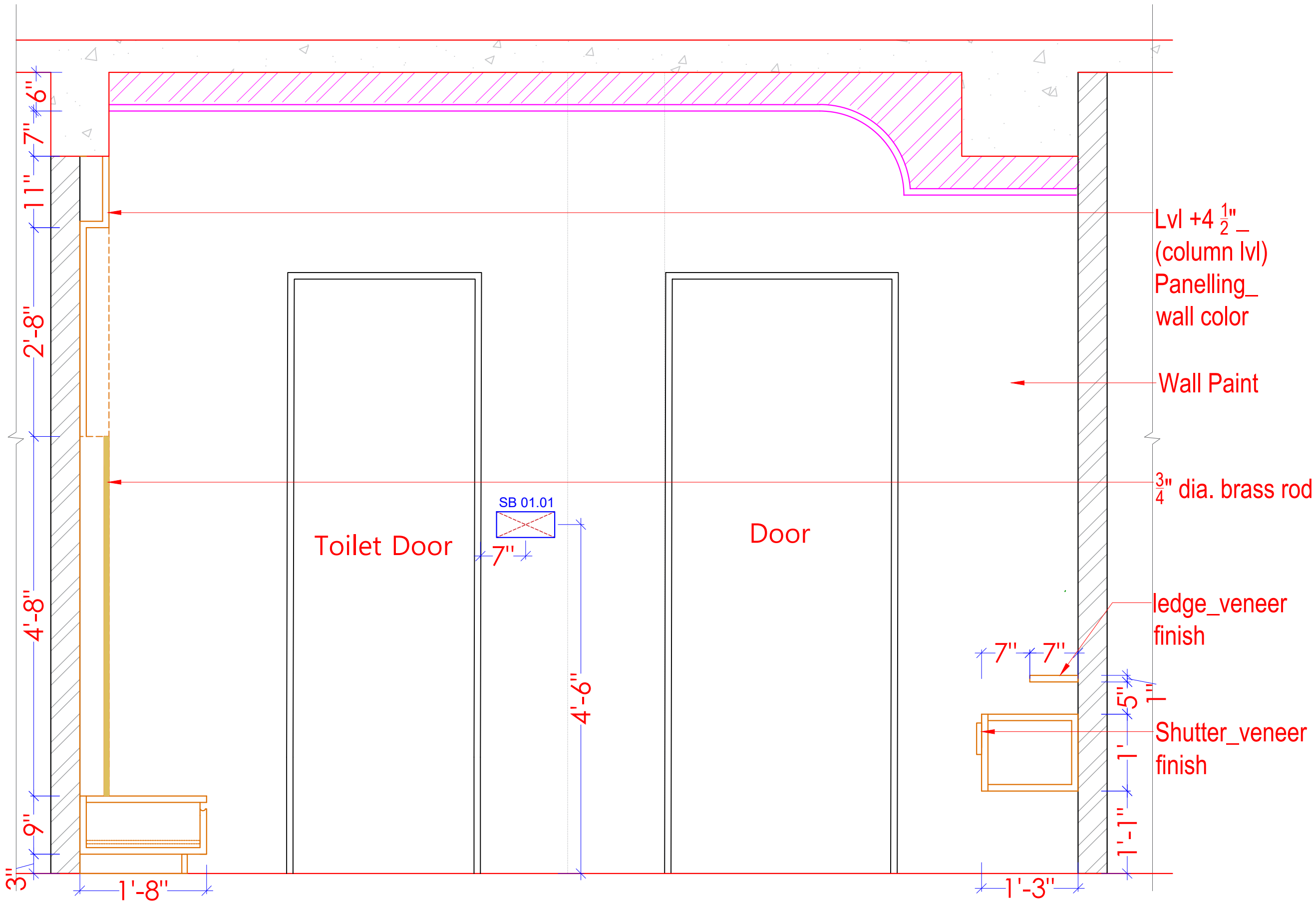
ELEVATION - D
