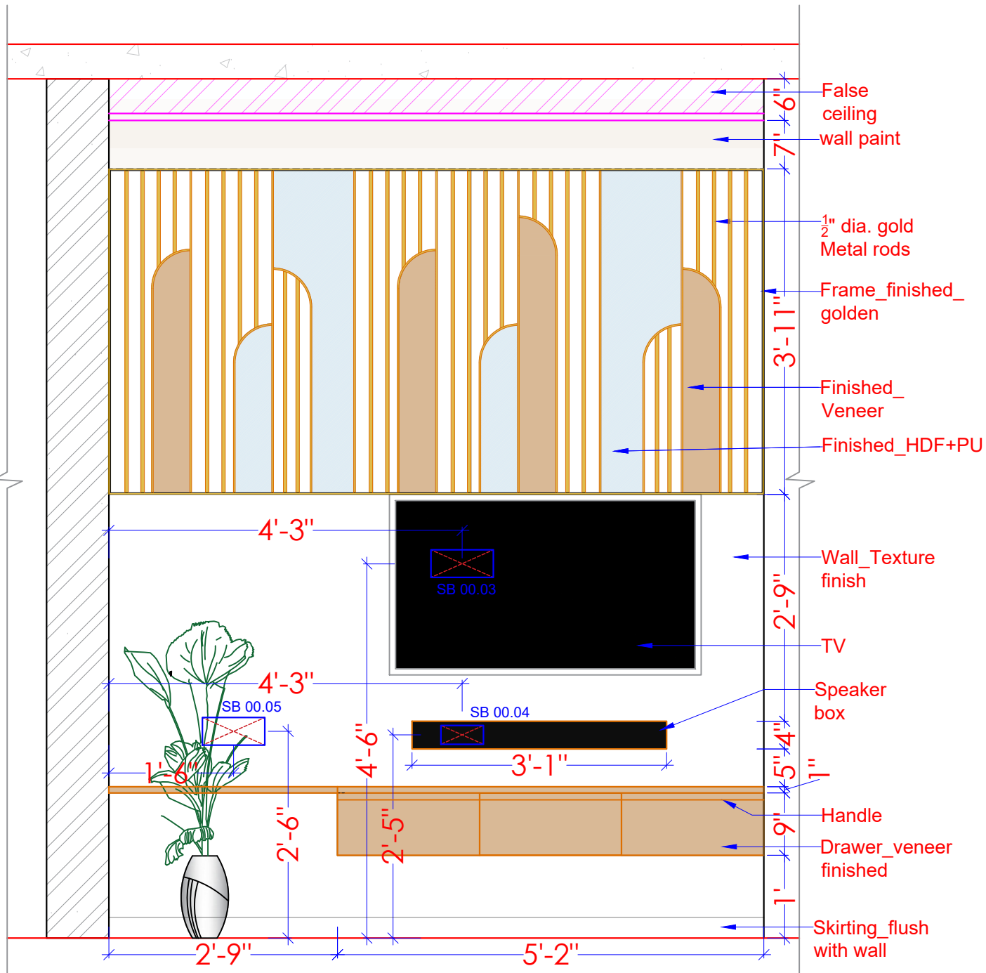
ELEVATION - A
