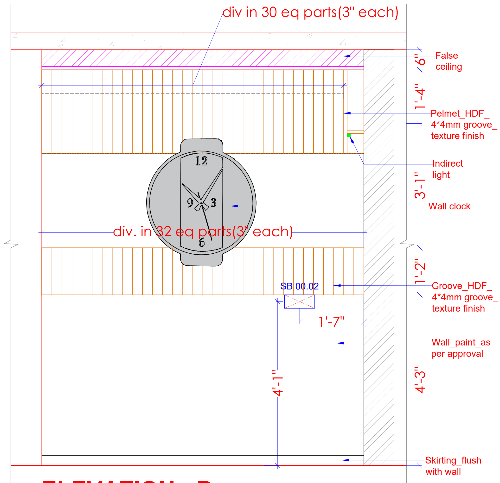
ELEVATION - B
