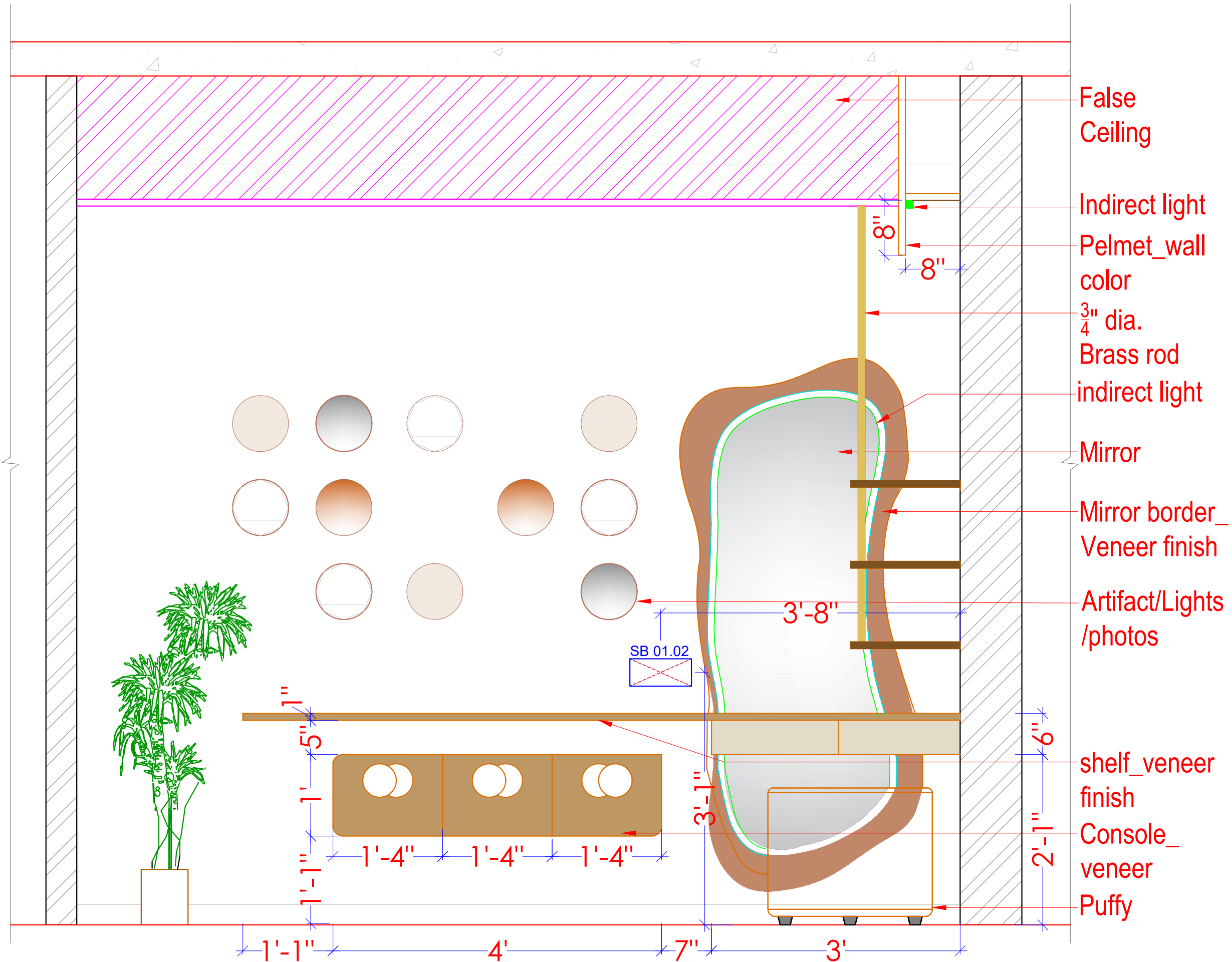
ELEVATION - A
